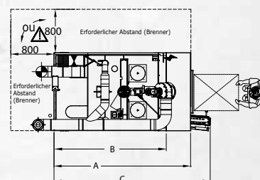
Seitenansicht
