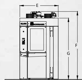
Frontansicht
