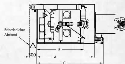
Seitenansicht
