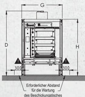
VORDERANSICHT MIT INTEGRIERTEN BESCHICKUNGSTISCH
