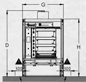
VORDERANSICHT MIT INTEGRIERTEN BESCHICKUNGSTISCH
