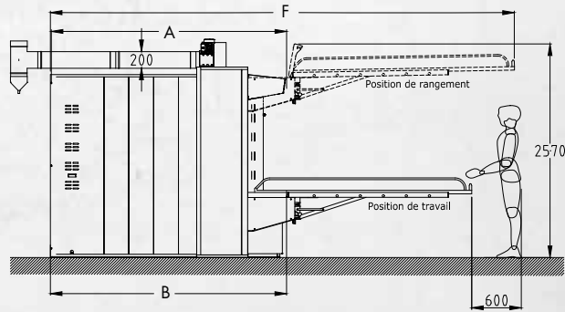
VUE LATERALE AVEC ELEVATEUR INTEGRE
