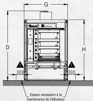
VUE DE FACE AVEC ELEVATEUR INTEGRE
