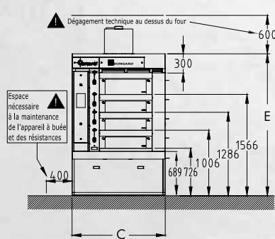
VUE DE FACE SANS ELEVATEUR INTEGRE
